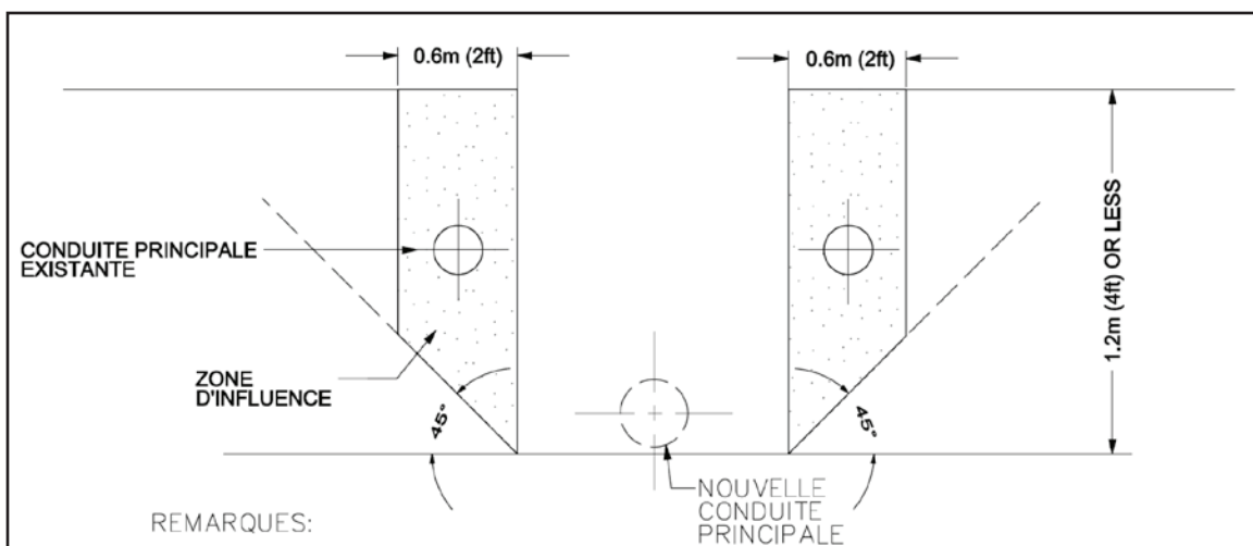
Figure 4-2 : Ligne d'influence pour les gazoducs parallèles aux excavations
